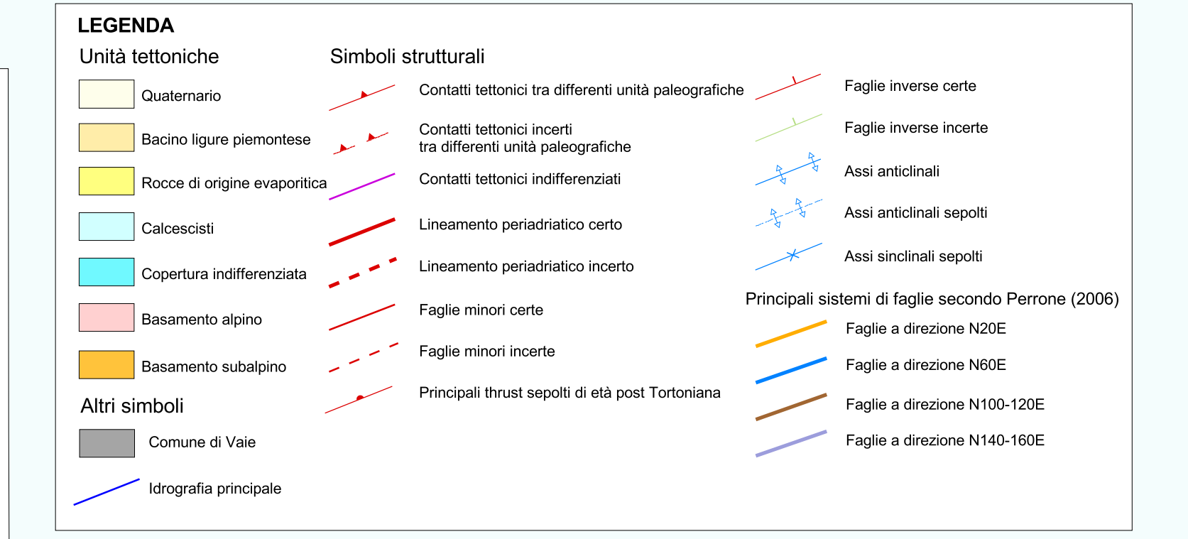
SCHEMA TETTONICO (modificato da Modello Strutturale d'Italia)
