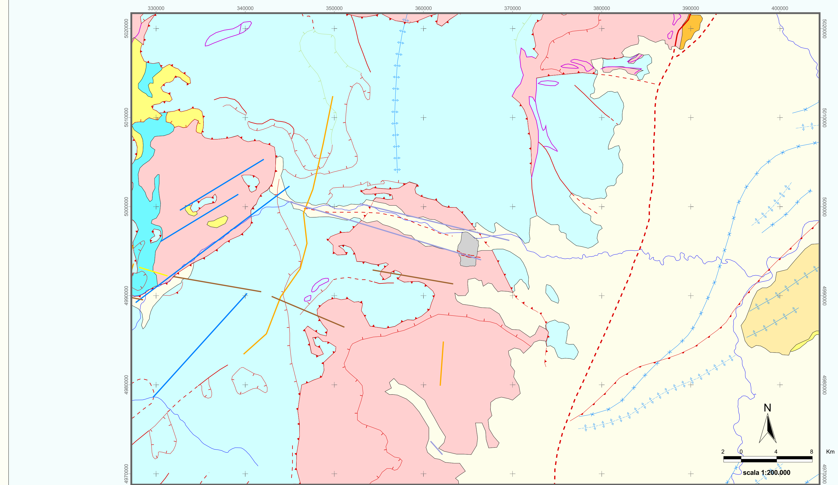
SCHEMA TETTONICO (modificato da Modello Strutturale d'Italia)
